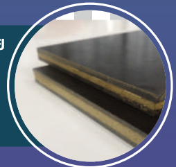
แผ่นไม้พลาสติกแซนวิชเสริมเส้นใย ธรรมชาติดูดซับเสียงและกรรม วิธีการผลิต คณะวิศวกรรมศาสตร์ มหาวิทยาลัยสงขลานครินทร์
